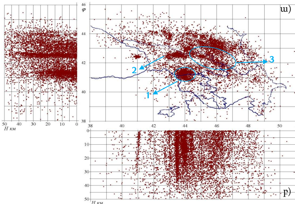
Նկ.5. Կովկասի 1971-2014թթ. երկրաշարժերի էպիկենտրոնների (ա) և հիպոկենտրոնների (բ) բաշխվածությունը վերահաշվարկից հետո
