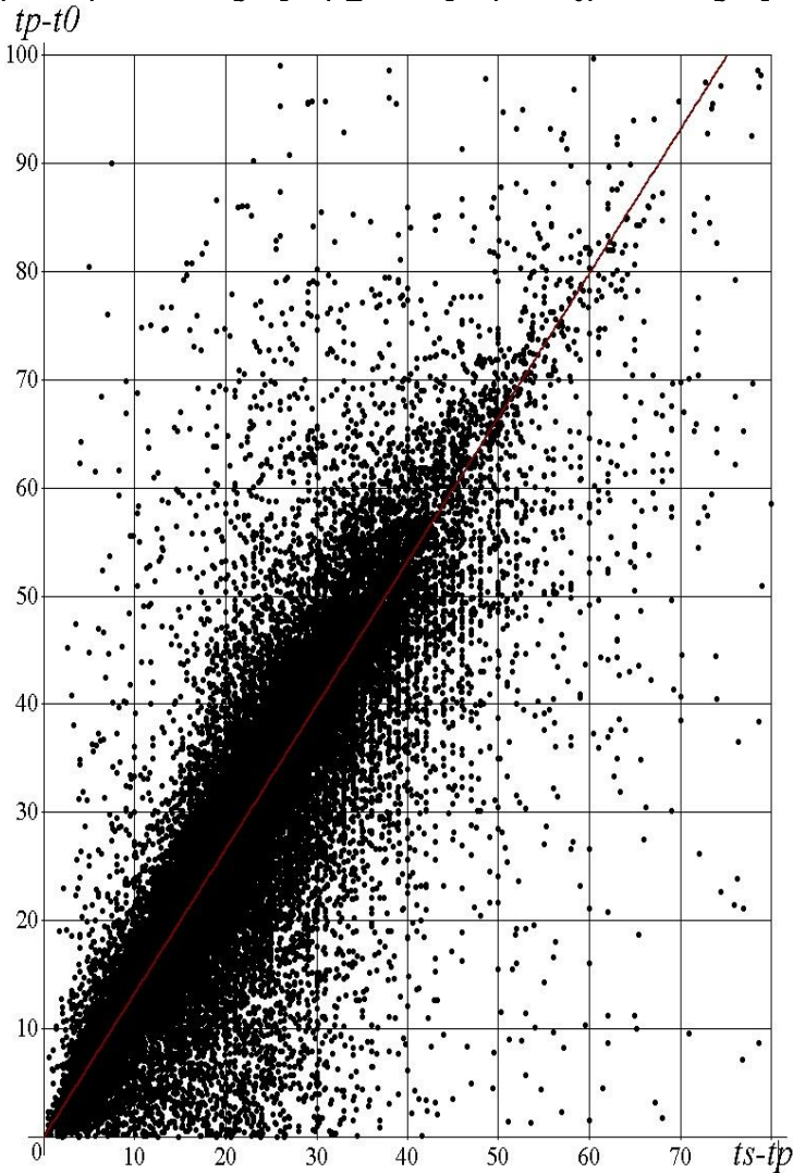
Նկ.1. Կովկասի երկրաշարժերի բյուլետենների տվյալներով ստացված Վադատիի գրաֆիկը
