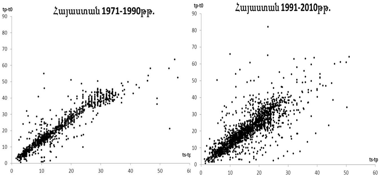
Նկ.2. Հայաստանի տարածքի 1971-1990թթ. և 1991-2010թթ. ժամանակահատվածների երկրաշարժերի բյուլետենների տվյալներով կառուցված Վադատիի գրաֆիկը
