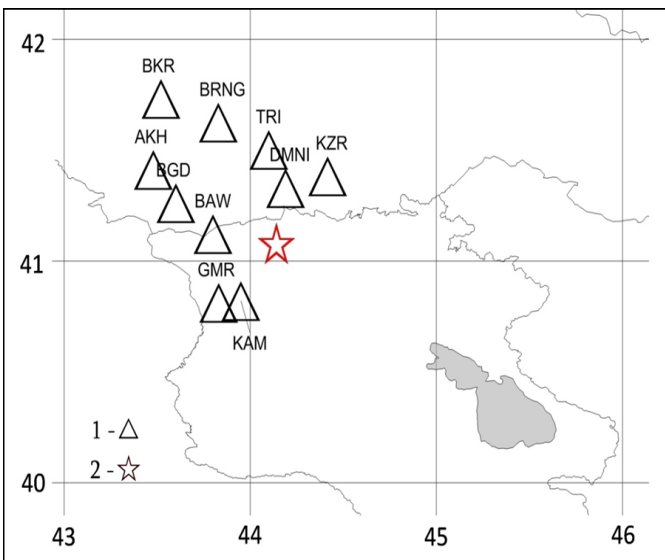
Նկ.7. Երկրաշարժի թեստային էպիկենտրոնը և գրանցած սեյսմիկ կայանները 1-սեյսմիկ կայանները, 2-երկրաշարժի էպիկենտրոնը
